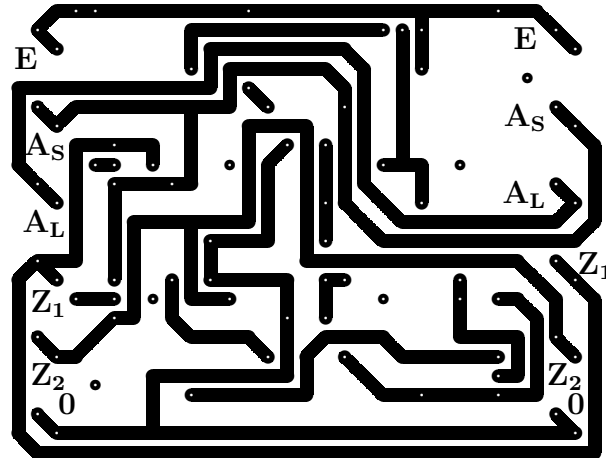
Abbildung 2.2: Ansicht von unten
