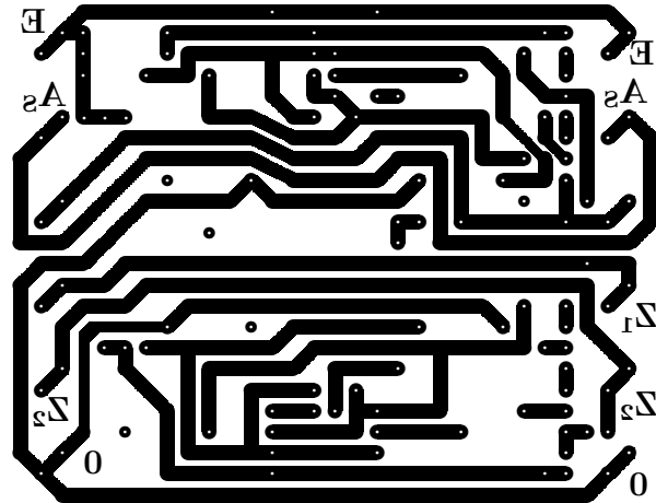
Abbildung 3.2: Aufsicht mit durchsichtiger Platine
