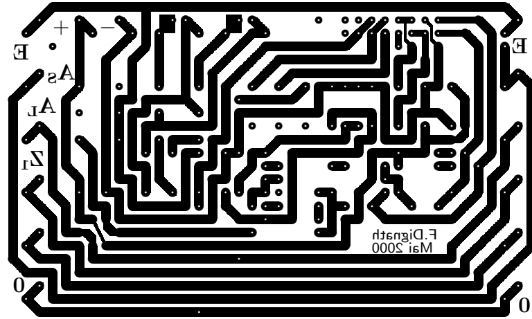
Abbildung 1.2: Ansicht von oben
