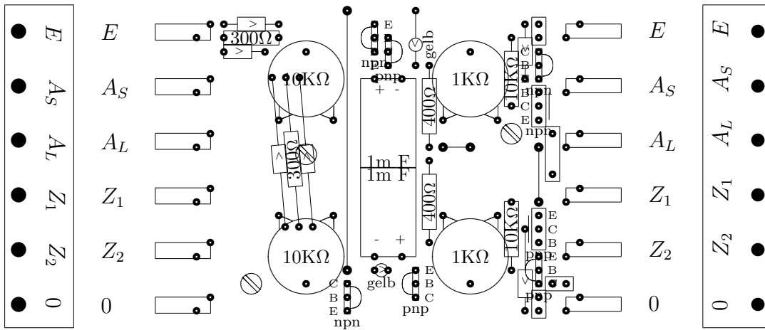
Abbildung 3.3: Ansicht von oben
