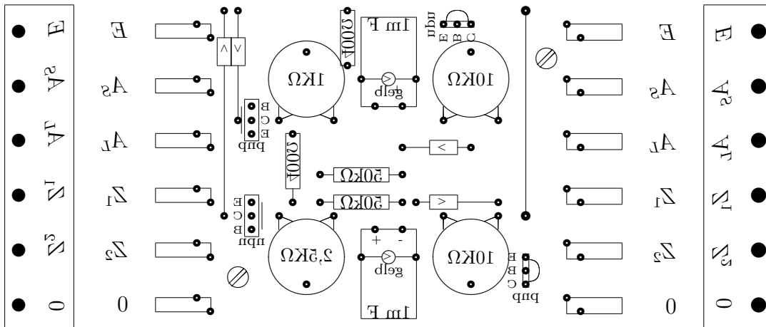
Abbildung 2.3: Ansicht von unten mit durchsichtiger Platine
