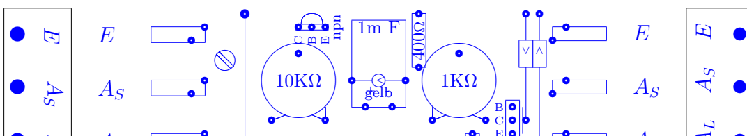
Abbildung 2.4: Ansicht von oben mit durchsichtiger Platine
