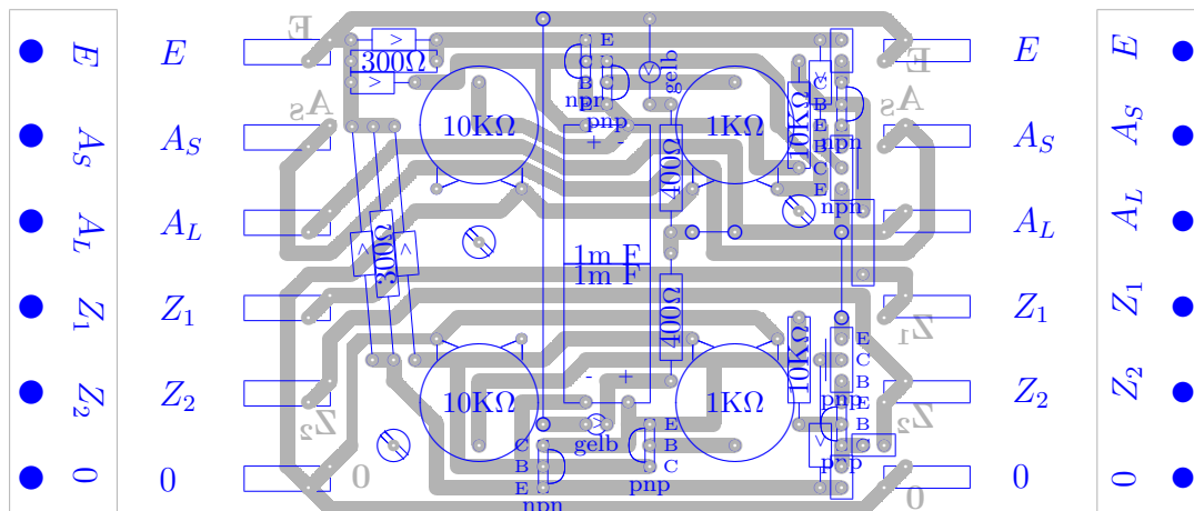
Abbildung 3.1: Aufsicht mit durchsichtiger Platine
