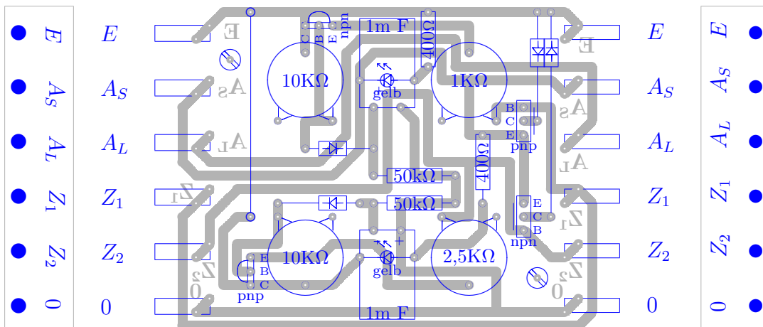
Abbildung 2.1: Aufsicht mit durchsichtiger Platine
