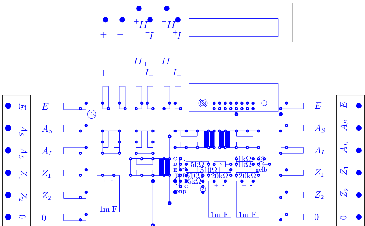
Abbildung 1.3: Ansicht von oben
