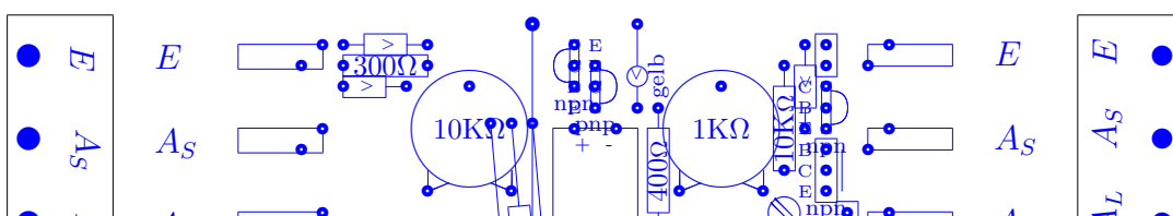
Abbildung 3.4: Ansicht von oben mit durchsichtiger Platine
